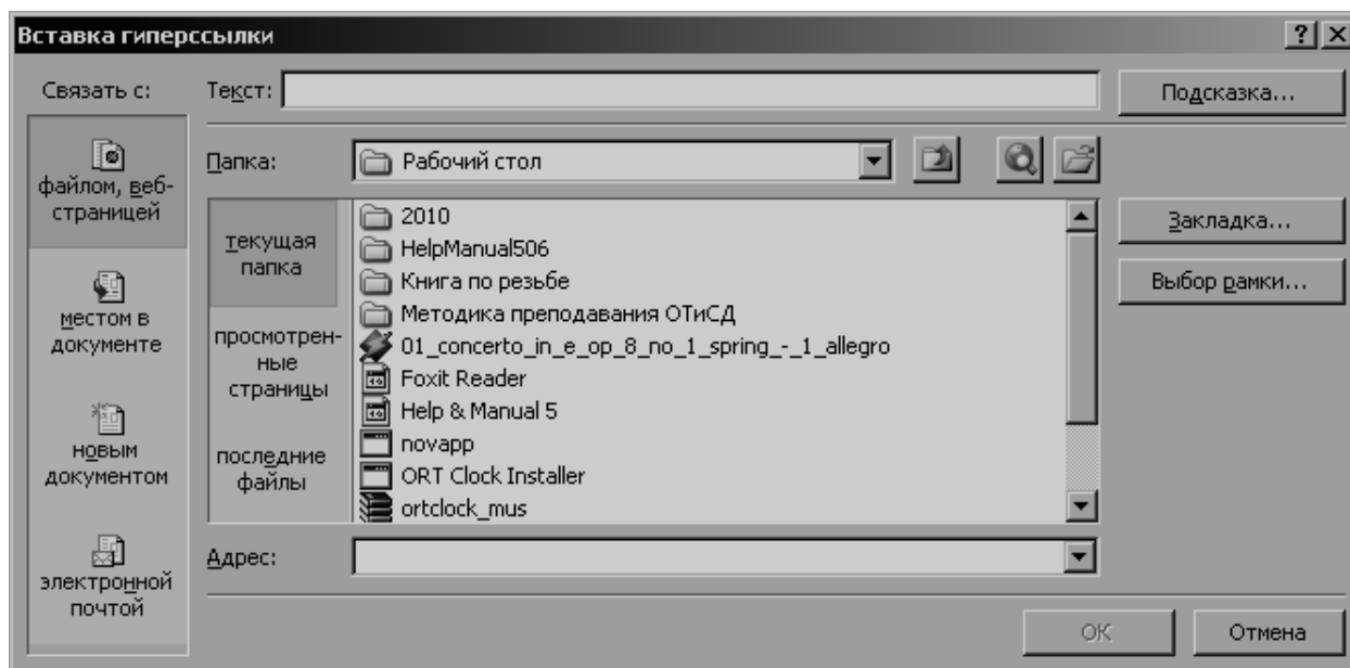
Рисунок 5.3 – Вставка гиперссылки
