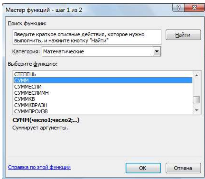
Рис. 6. Мастер функций
