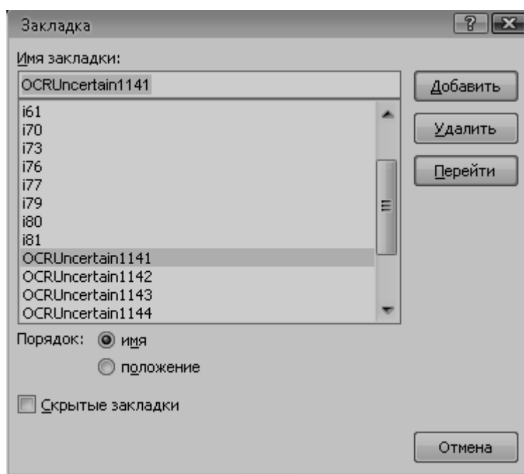
Рисунок 5.1 – Вставка закладки
