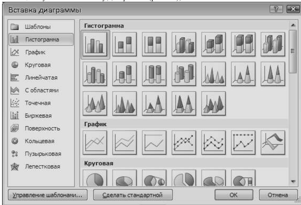
Рисунок 6.5 – Вставка диаграммы
