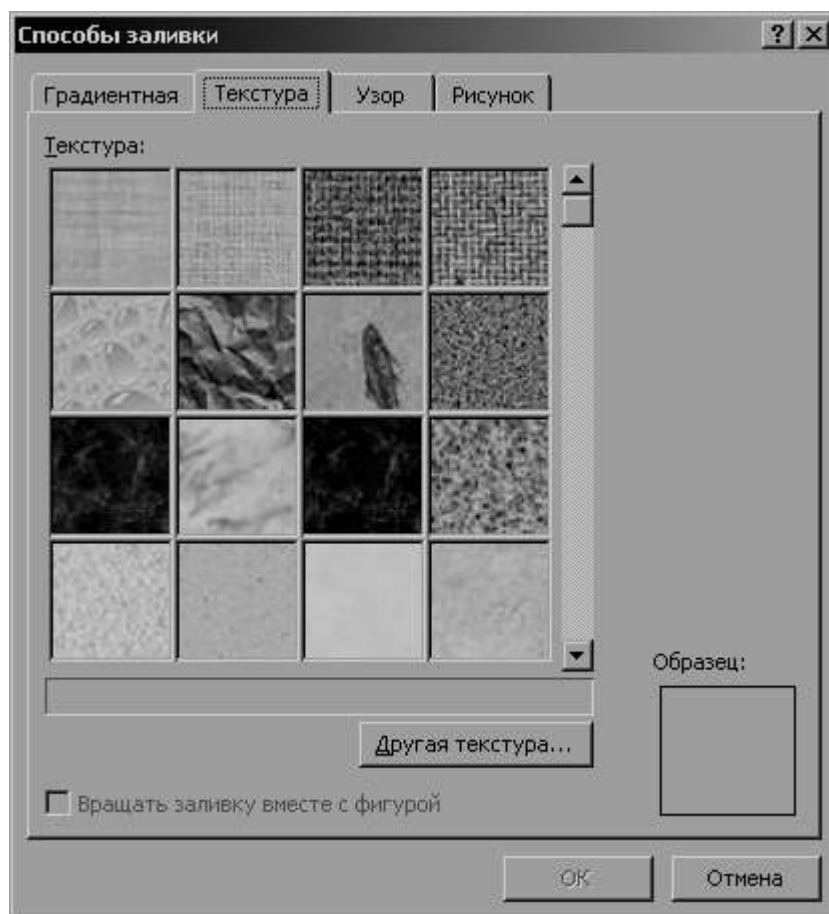
Рисунок 5.2 – Выбор текстуры
