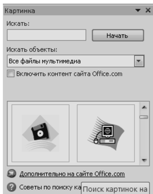
Рисунок 6.5 – Вставка картинки
