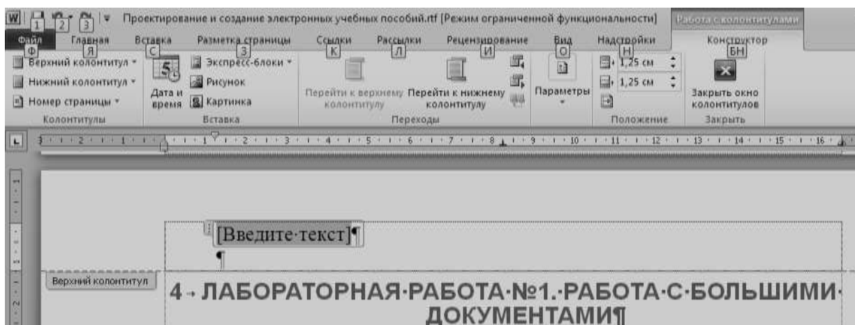
Рисунок 4.1 – Редактирование колонтитулов
