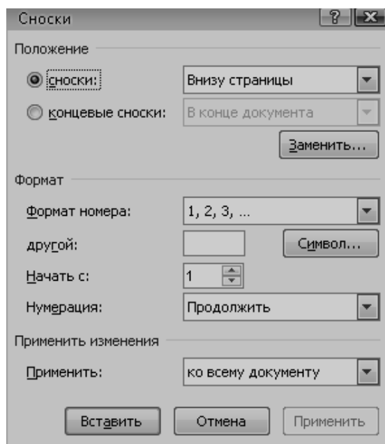
Рисунок 4.2 – Вставка сносок
