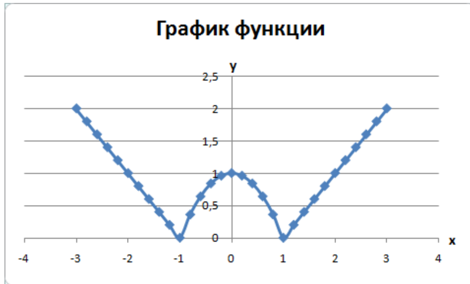
Рис. 12. График функции
