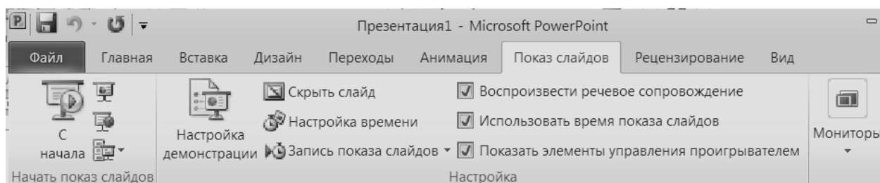
Рисунок 6.6 – Показ слайдов
